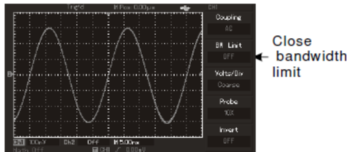
Fig. 2-5 Fara limitarea benzii semnalului de intrare
