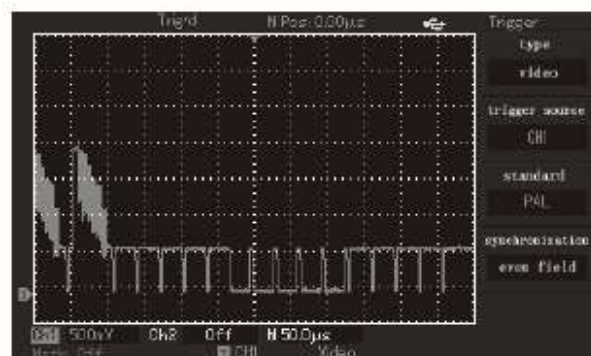
Fig. 2-15 Video trigger: sincronizare pe camp
