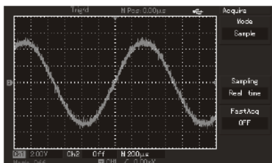
Fig. 2-19 Semnal fara mediere
