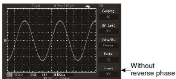
Fig. 2-8 Fara inversare faza
