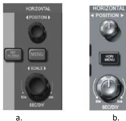
Fig. 1-10 Control orizontal osciloscop: a. ecran de 5.7 inch b. ecran de 7 inch
