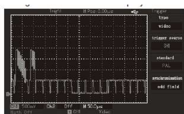
Fig. 3-8 Semnal video campuri
