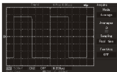
Fig. 3-5 Semnalul de intrare “curatat” de zgomot
