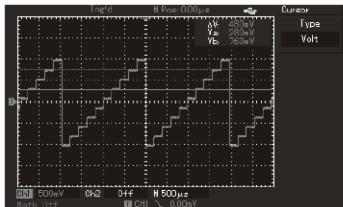
Fig. 3-6 Masurarea treptei de tensiune cu ajutorul cursorului
