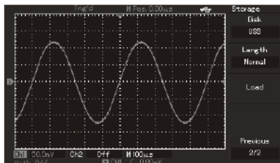
Fig. 2-24 Inregistrare forma de unda prin U disk
