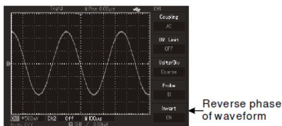
Fig. 2-9 Cu inversare faza
