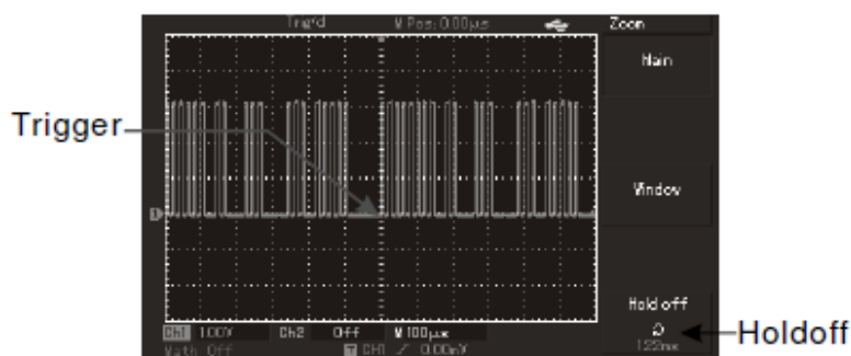
Fig. 2-17 Utilizarea timpului de retinere
