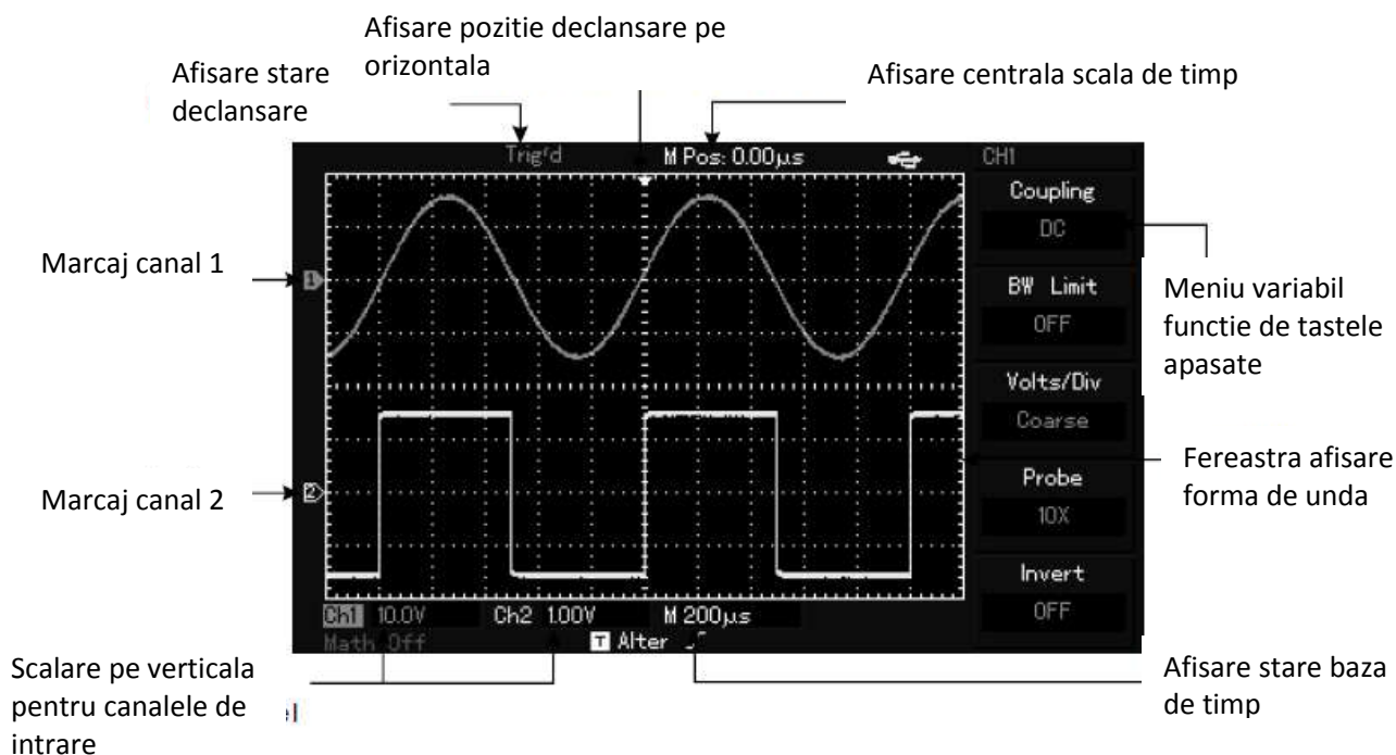
Fig. 1-3 Interfata afisaj (pentru osciloscoapele din familia UTD2000L)
