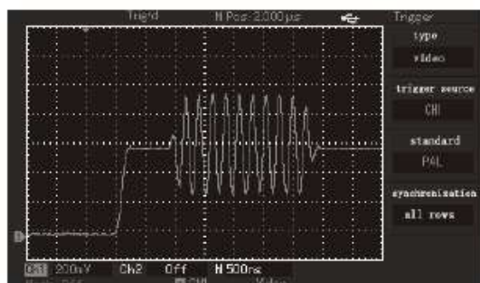
Fig. 2-14 Video trigger: sincronizare pe linie
