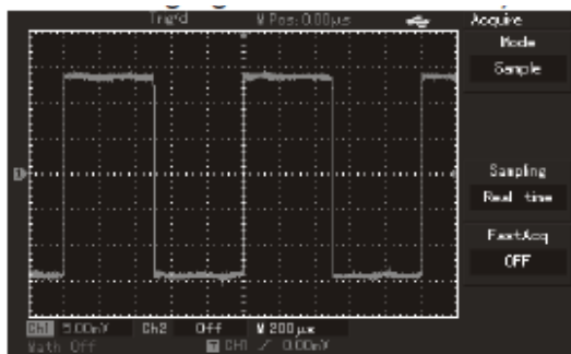
Fig. 3-4 Semnal de intrare “zgomotos”
