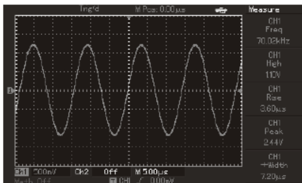
Fig. 3-1 Masurare automata a unui semnal simplu
