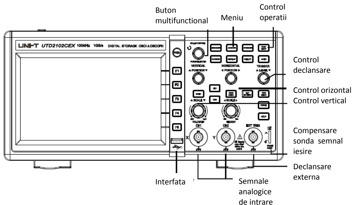
Fig. 1-2 Configuratia panoului frontal a ecranului LCD de 7 inch.
