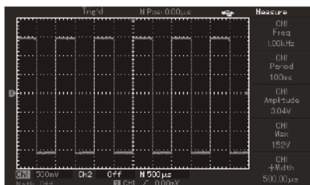
Fig. 3-15 Copiere ecran
