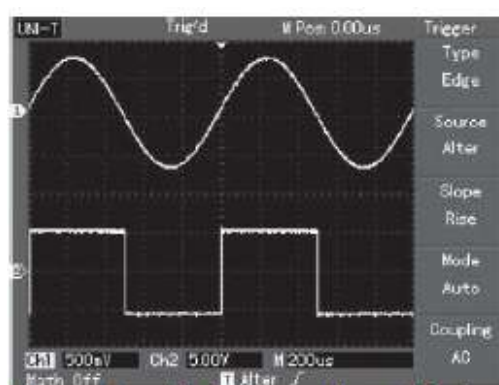
Fig. 2-16 Observarea simultana a 2 semnale diferite
