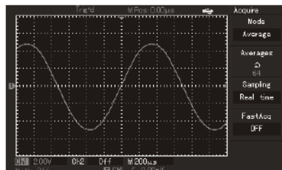
Fig. 2-20 Semnal cu mediere 32 (32 esantioane mediate)
