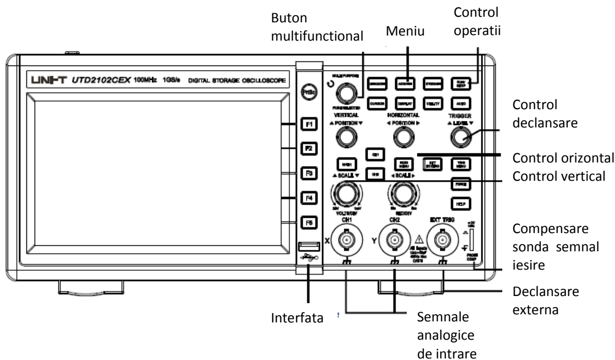
Fig. 1-2 Configurația panoului frontal a ecranului LCD de 7 inch.
