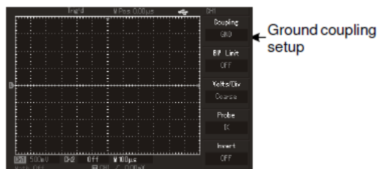
Fig. 2-3 Cuplare "grounding"
