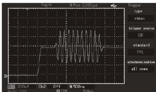
Fig. 2-14 Video trigger: sincronizare pe linie
