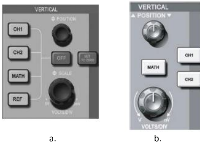
a. b. Fig. 1-9 Control vertical osciloscop: a. ecran de 5.7 inch b. ecran de 7 inch
