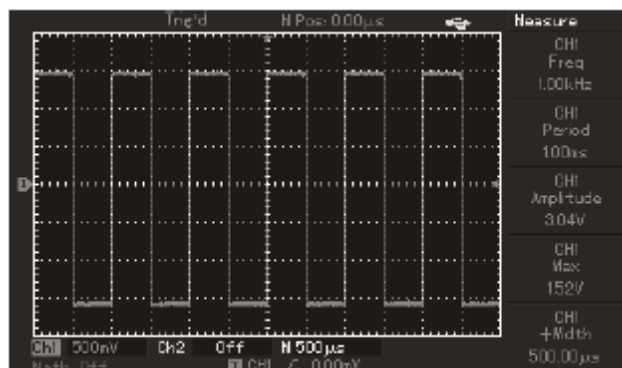
Fig. 3-15 Copiere ecran
