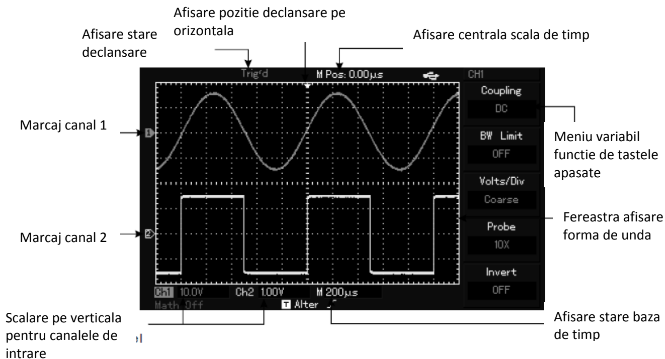
Fig. 1-3 Interfața afisaj (pentru osciloscoapele din familia UTD2000L)
